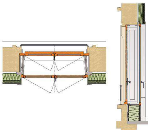
▲ Figure 8 Exemple de double fenêtre mise en œuvre côté intérieur avec isolation thermique intérieure complémentaire. Réalisation à Lyon
