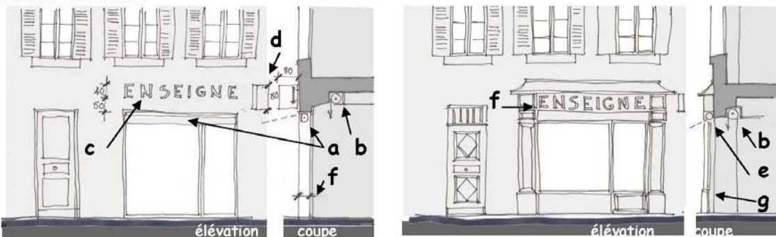
VITRINE EN FEUILLURE dans baie rectangulaire (B)
