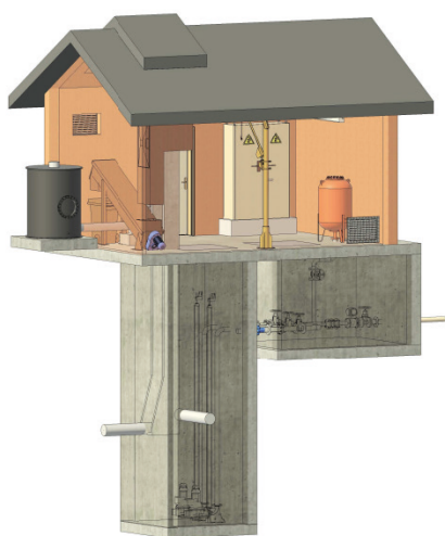
Schéma du poste de relèvement « principe PR87 »
