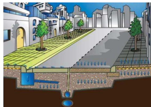
Chaussée à structure réservoir
